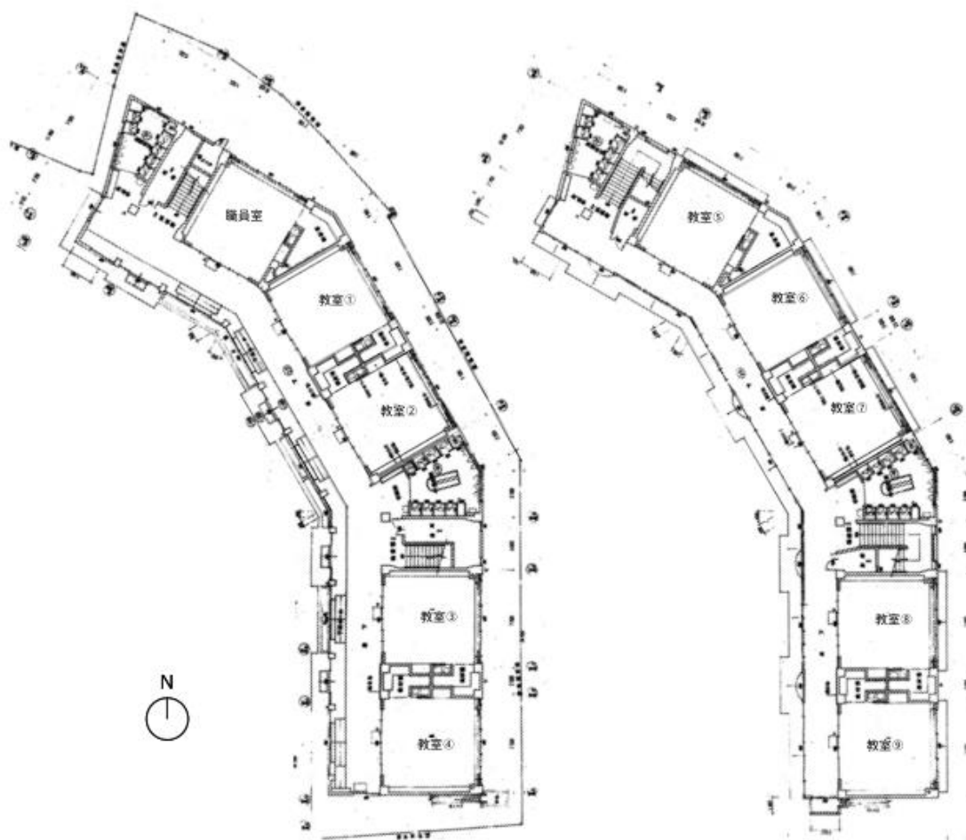
1F平面図 1/450
