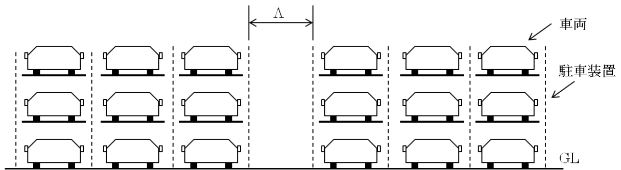
(断面図)
