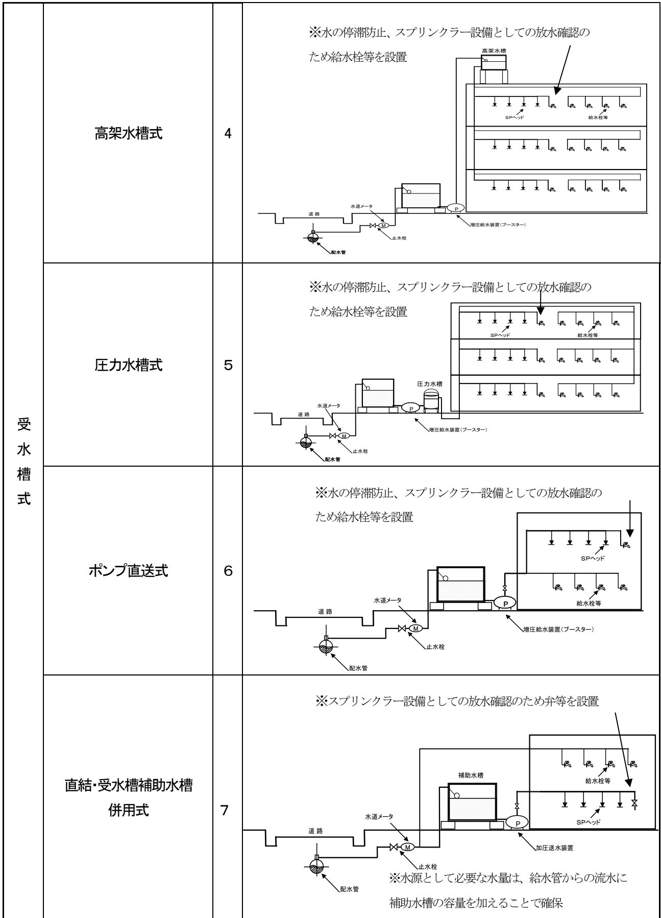
第4-33図 特定施設水道連結型スプリンクラー設備の給水方式
