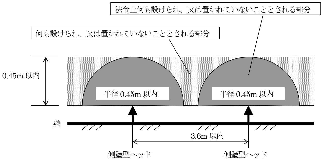
第 4-14 図 側壁型ヘッドの設置
