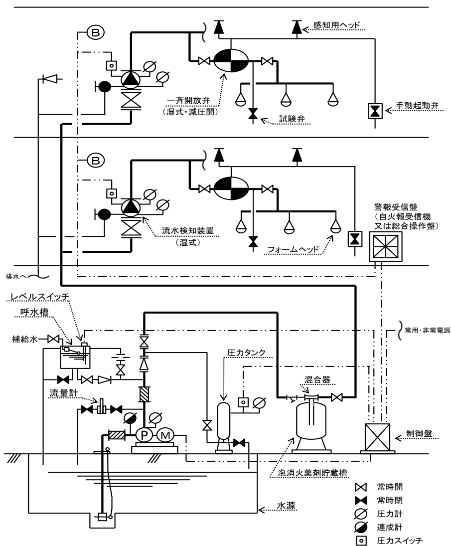
第6-1図 泡消火設備の構成・系統図例（プレッシャー・プロポーショナル方式）
